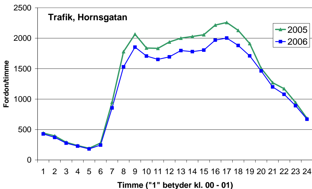
Figur 13. Genomsnittliga variationer av trafikflöden under vardagsdygnet (måndagar – torsdagar) under januari – april år 2005 och 2006 vid Hornsgatans fasta mätstation.
