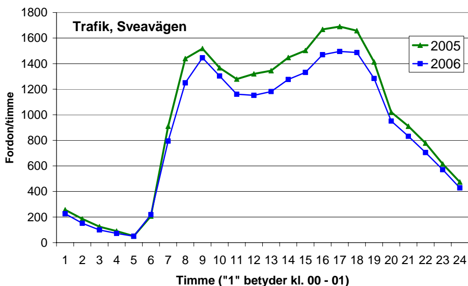
Figur 15. Genomsnittliga variationer av trafikflöden under vardagsdygnet (måndagar – torsdagar) under januari – april år 2005 och 2006 på Sveavägen (mellan Adolf Fredriks Kyrkogata och Kammakargatan).
